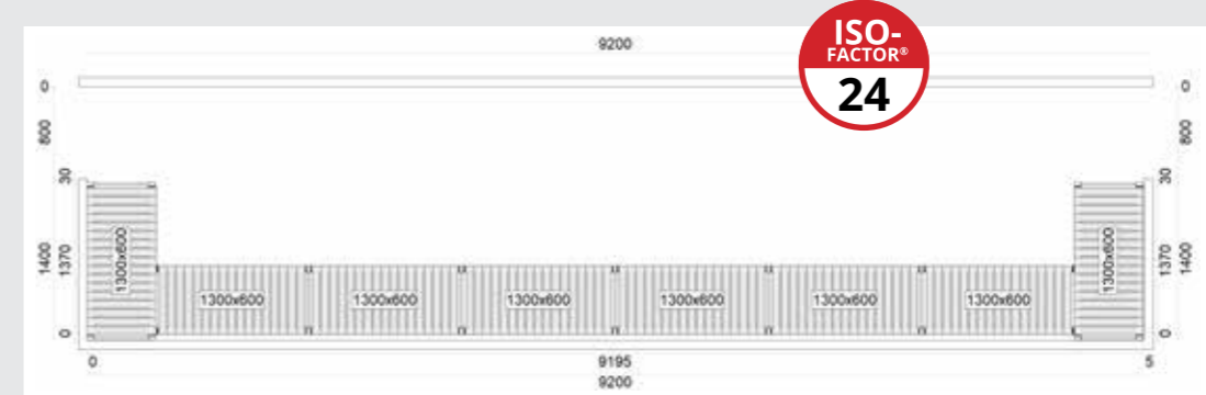
Lager indrettet med statiske enheder
