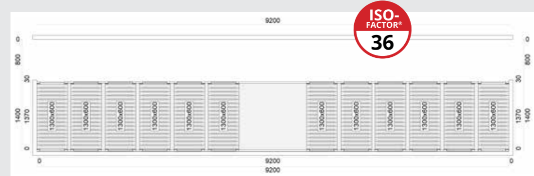
Lager indrettet med mobile enheder
